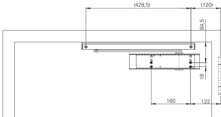
mit Montageplatte / with mounting plate / avec plaque de montage
